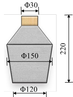
图 10 坛状砝码 (单位: mm)
